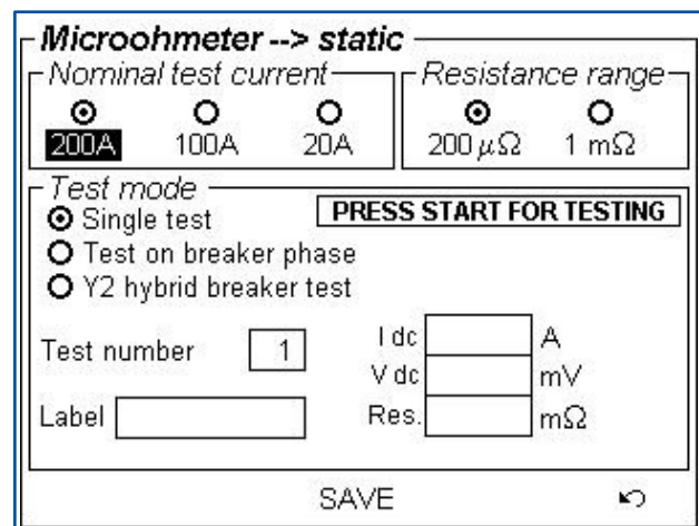
Microohmmeter display
